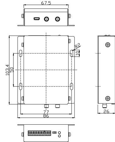
Габаритные размеры(мм)
